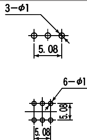
取付穴参考寸法 Mounting Hole
